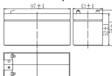
Габариты
