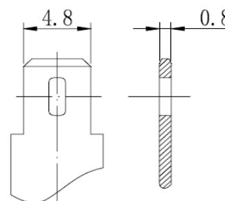
Позиция клемм
